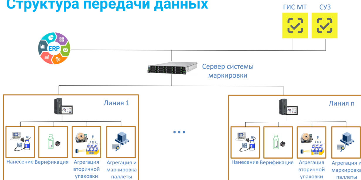
Рисунок 1. Общая схема работы системы АСПУ
