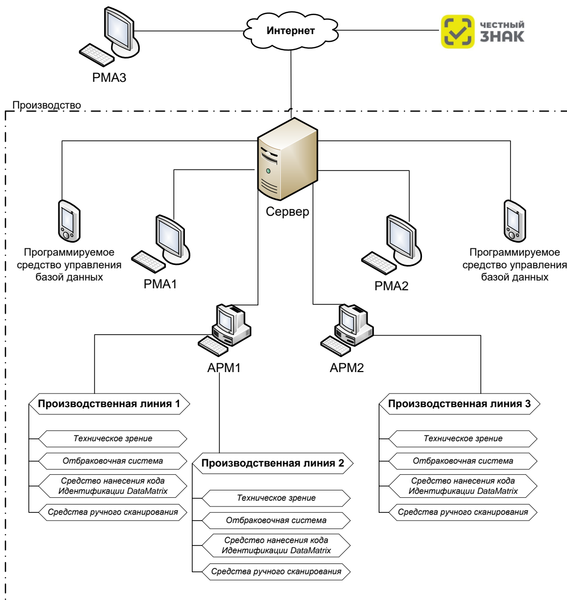
Общая структурная схема системы
