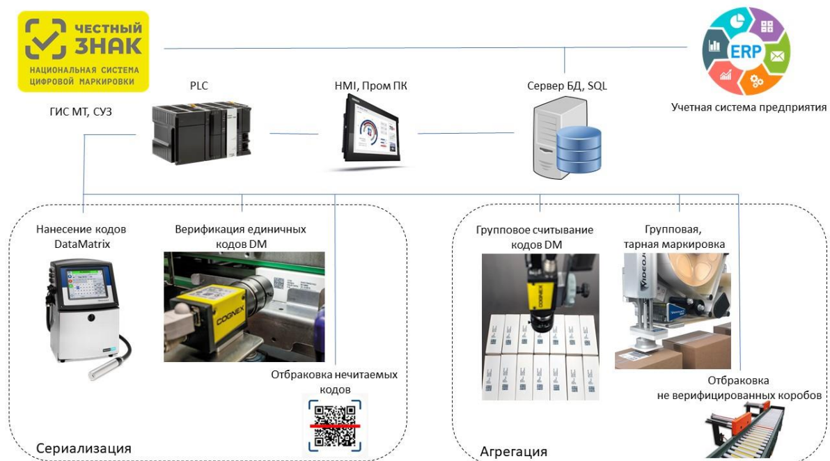
Рис. 1 Общая схема
