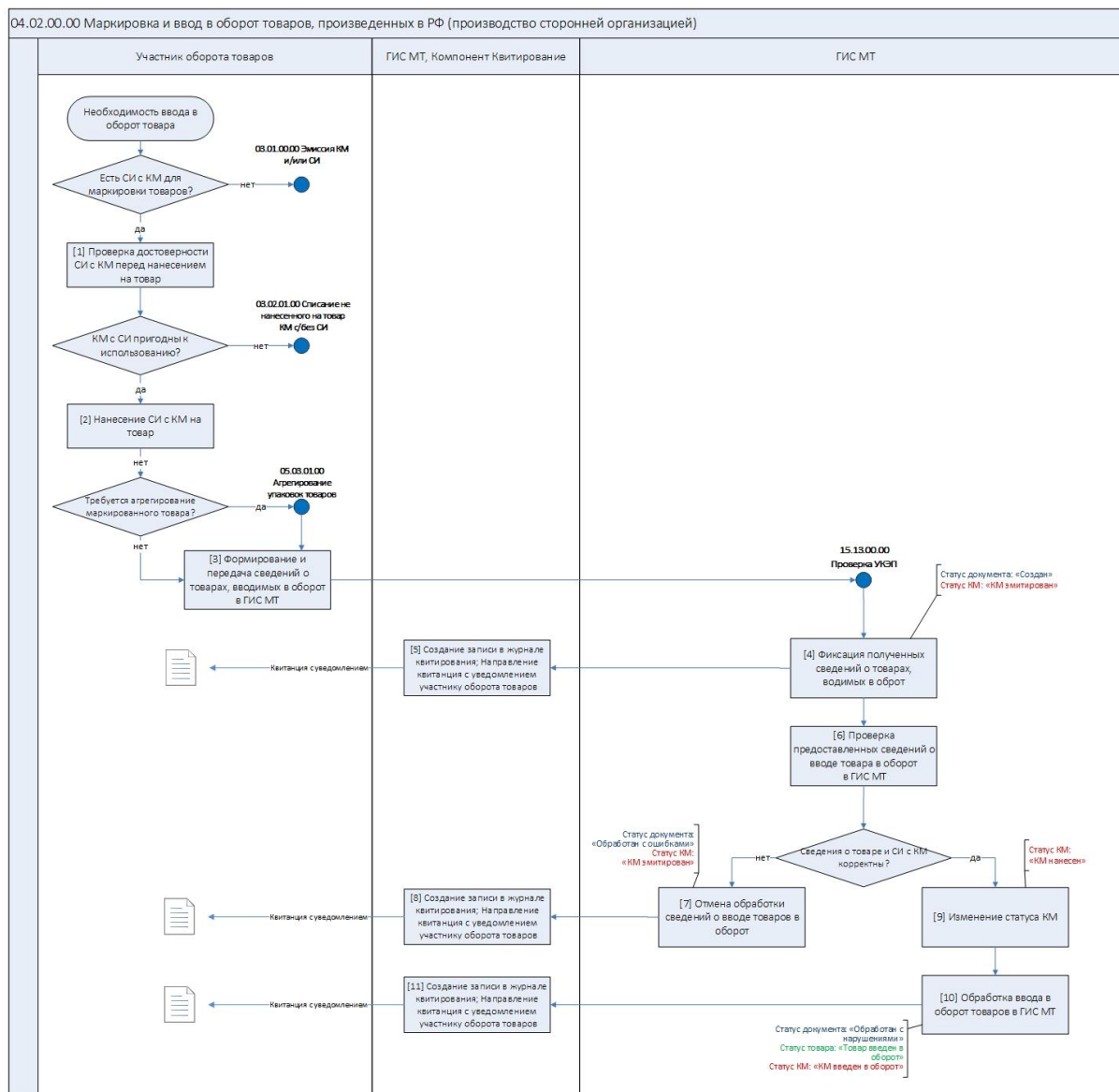
Рисунок 1 Схема процесса 04.02.00.00 Маркировка и ввод в оборот шин, произведенных в РФ (производство сторонней организацией)
