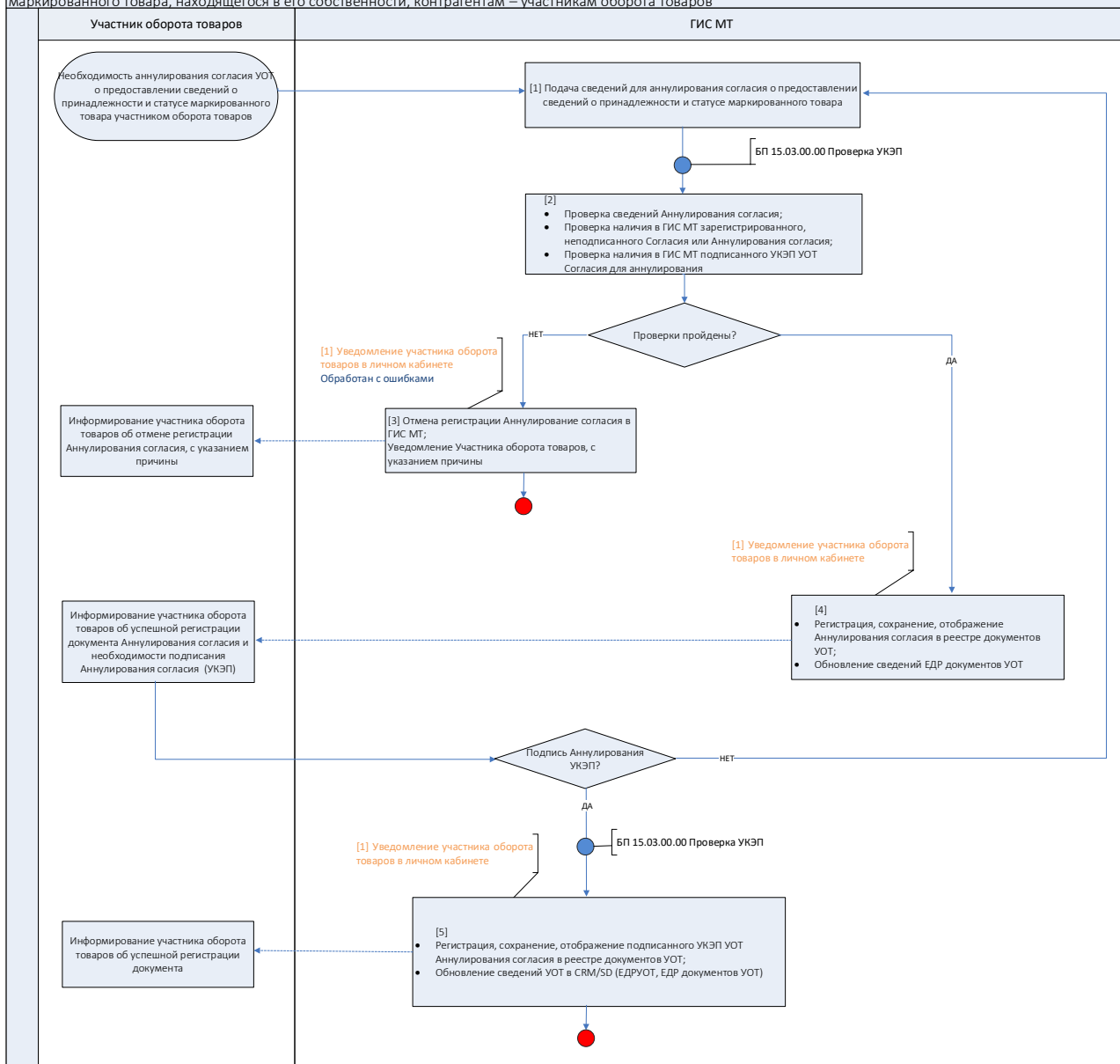
Рисунок 2 Схема процесса 05.01.08.02 Аннулирование предоставленного в ГИС МТ согласия Участником оборота товаров о предоставлении информации о принадлежности и статусе маркированного товара в ГИС МТ, находящегося в его собственности, контрагентам – участникам оборота товаров
