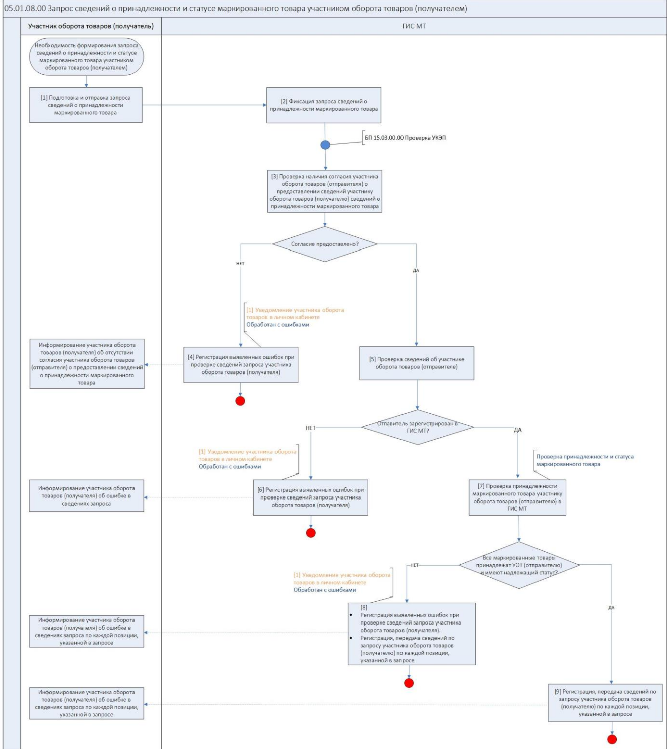
Рисунок 3 05.01.08.00 Запрос сведений о принадлежности и статусе маркированного товара участником оборота товаров (получателем)
