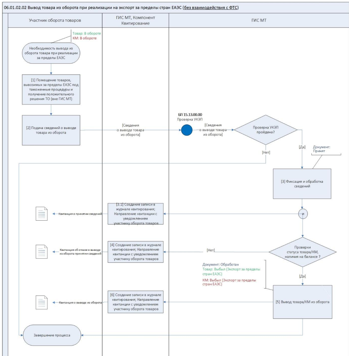
Рисунок 1 Схема процесса 06.01.02.02 Вывод товара из оборота при реализации товаров в страны, не являющиеся членами ЕАЭС
