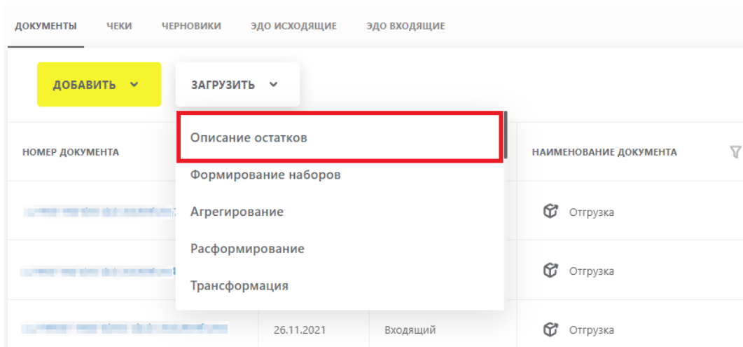
Рисунок 9. Загрузка документа
