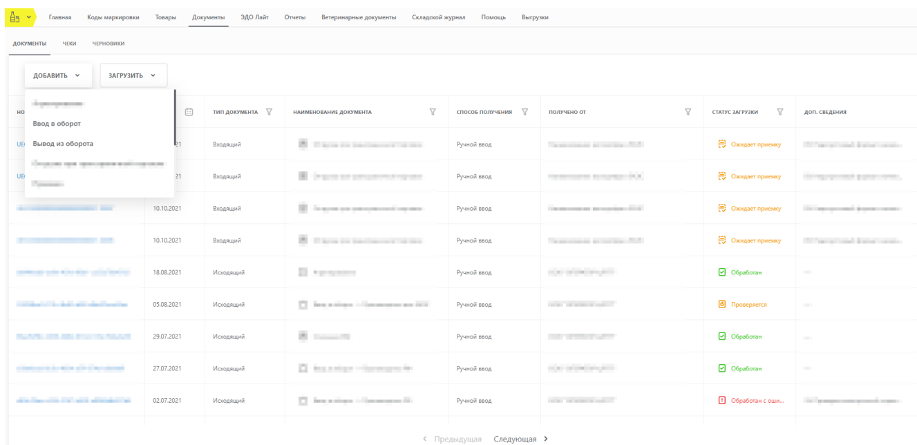
Рисунок 2. Добавление документа
