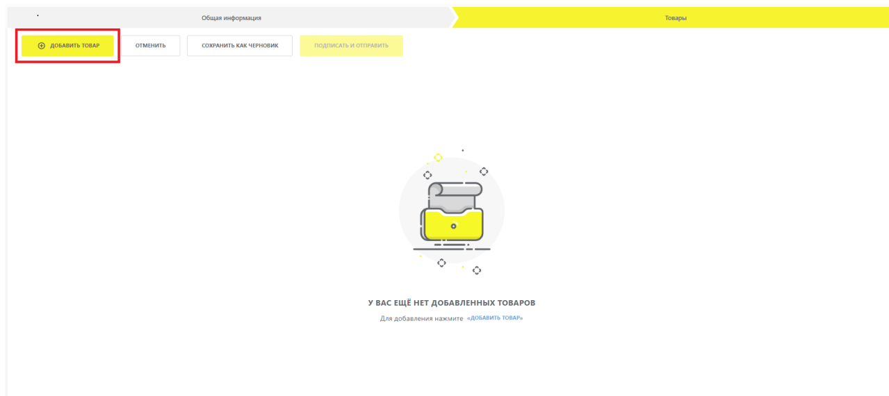
Рисунок 10. Товары
