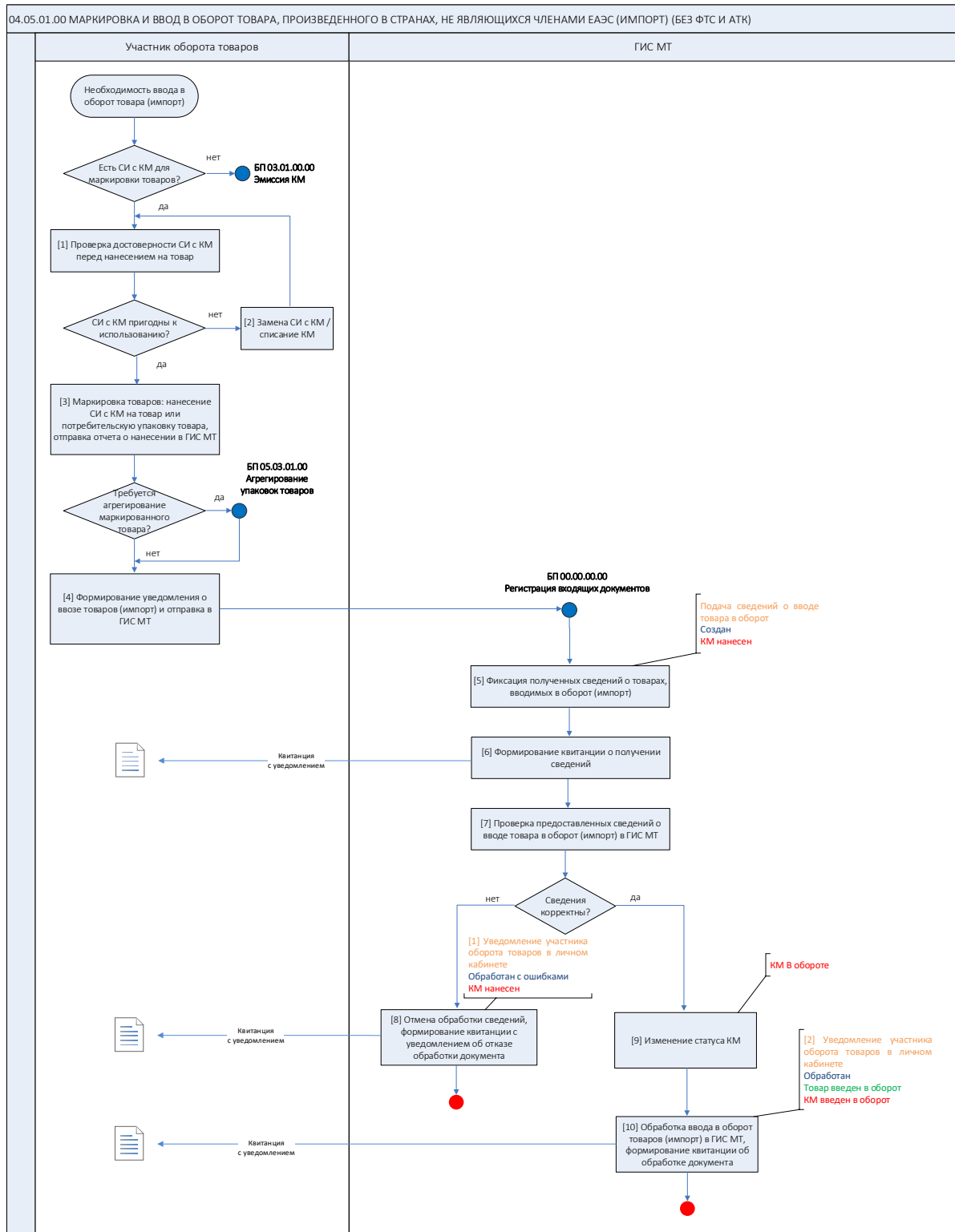
Рисунок 1 Схема процесса 04.05.01.00 Маркировка и ввод в оборот товара, произведенного в странах, не являющихся членами ЕАЭС (импорт) (без ФТС и АТК)
