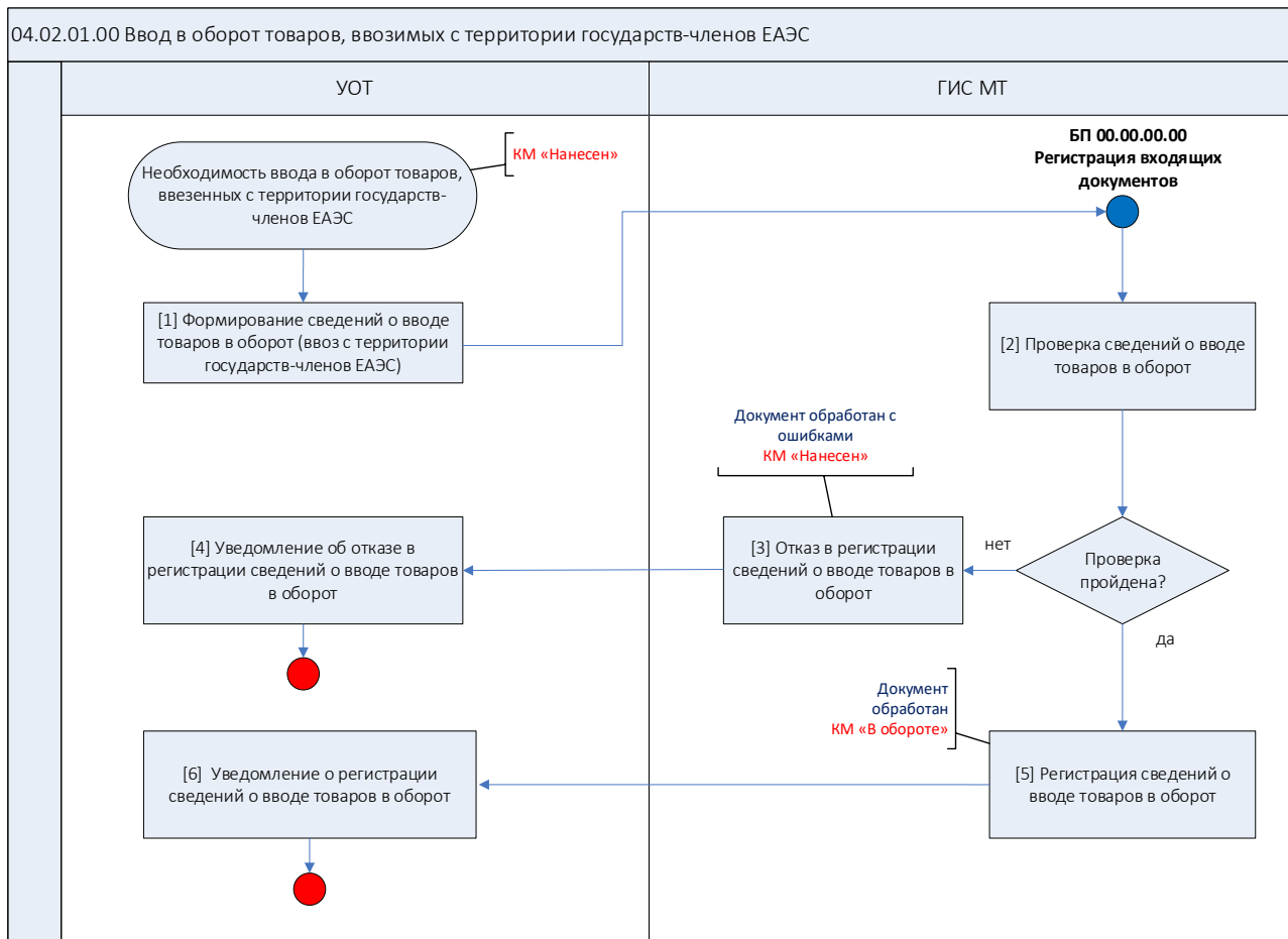
Рисунок 1 Схема процесса 04.02.01.00 Ввод в оборот товаров, ввезенных с территории государств-членов ЕАЭС
